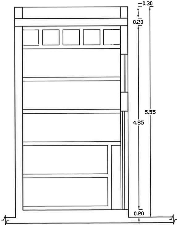
Sezione Trasversale
