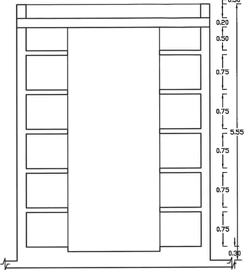
Sezione Longitudinale
