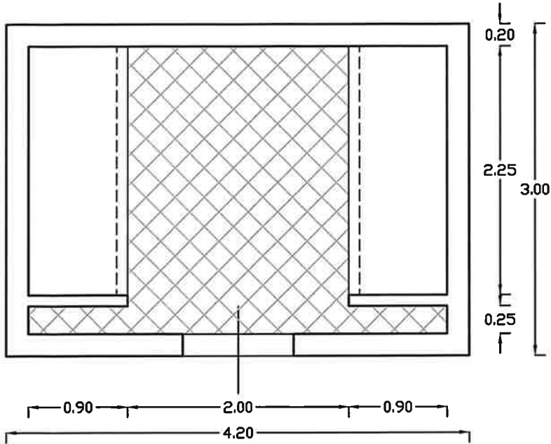
Pianta Quota 2.30
