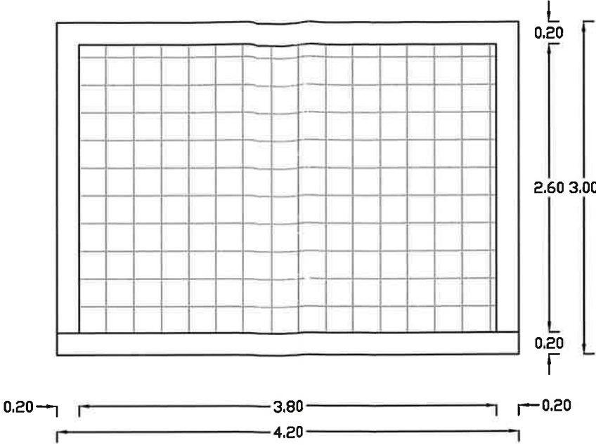
Pianta Quota 5.60
